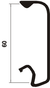
PG 145 Bagueta Omega 60 mm
