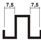
ES 150 Galley for 7,5 mm
