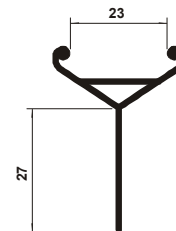
TB 427 Pipe Holder Y
