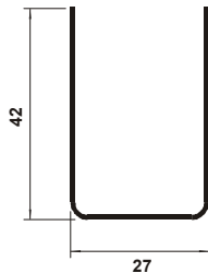
TB 419 Edge U for 25 mm
