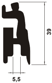
TB 307 Edge "J" for 13 mm
