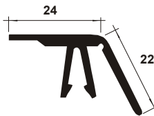
PV 392 Clip for Swing Door
