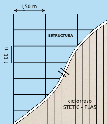
VISTA CON ESTRUCTURA
