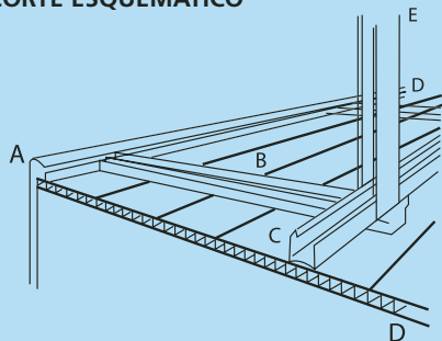
CORTE ESQUEMATICO
