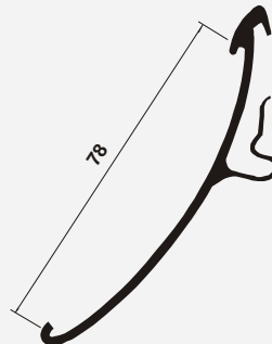
PP 157 Portaprecios Coextrusión c/Enganche
