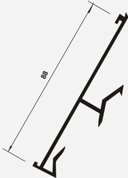
PP 153 Portaprecios Plano Grande Doble Sujeción
