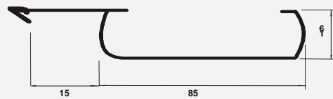
SP 085 Machimbre para Portador Metálico
