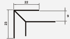
SP 102 Esquinero para 9 mm
