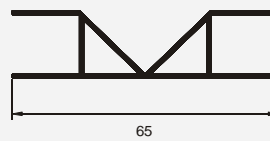
SP 209 Unión bisagra para 14,5 mm
