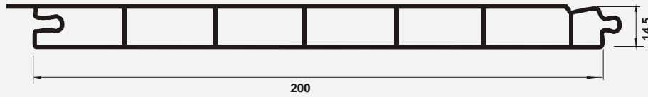
SP 200 Machimbre 200 mm
