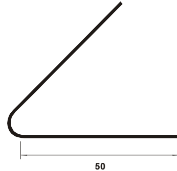
AN 211 Ângulo 50 esp. 2 mm
