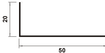
AN 214 Ângulo 50x20 esp.1 mm
