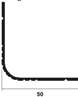
AN 213 Ângulo 50 estriado
