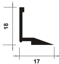
AN 216 Ângulo clip contravidrio
