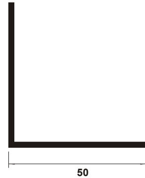
AN 211 Ângulo 50 esp. 2 mm
