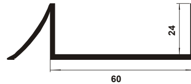
GU 361 Guia Painel para Câmara 60 mm
