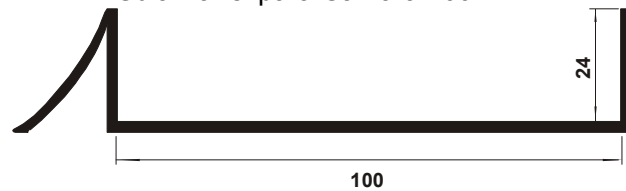
GU 362 Guia Panel para Câmara 100 mm
