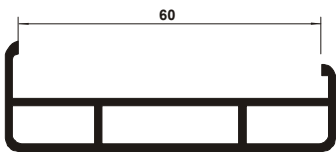
CL 437 Vão de Porta 60 mm
