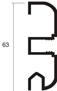
CL 478 Paragolpes Reto 63 mm
