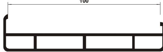
CL 438 Vão de Porta 100 mm
