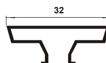
ES 151 Tampa Ranhura Painel
