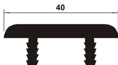
TC 100 Fitas de Borda 40 com Insertos
