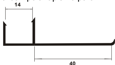
TB 434 Marco Apoia-lápis 40 para 14 mm TB 435 Marco Apoia-lápis 25 para 14 mm
