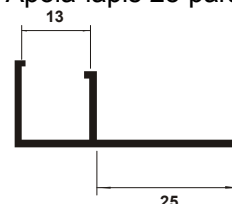
TB 431 Marco Apoia-lápis 25 para 7 mm TB 432 Marco Apoia-lápis 25 para 13 mm TB 433 Marco Apoia-lápis 25 para 13 mm
