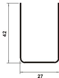
TB 419 Borda U para 25 mm
