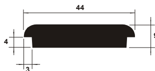
TC 101 Fitas de Borda 40 Maciço
