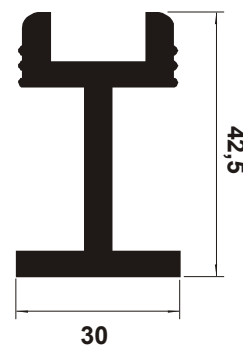
TB 361 Rodapé Duplo T
