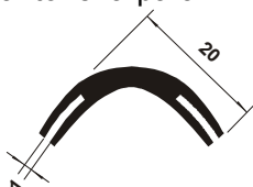
TB 444 Cantoneira para 1 mm
