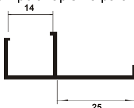
TB 434 Marco Apoia-lápis 40 para 14 mm TB 435 Marco Apoia-lápis 25 para 14 mm
