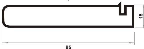
TB 449 Tubo 85 para Gaveta
