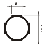
TO 027 Redondo Facetado 18,5
